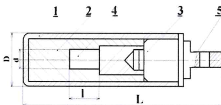
в) тип ГС75М13 (хвостовик капсулы с лопаткой)
