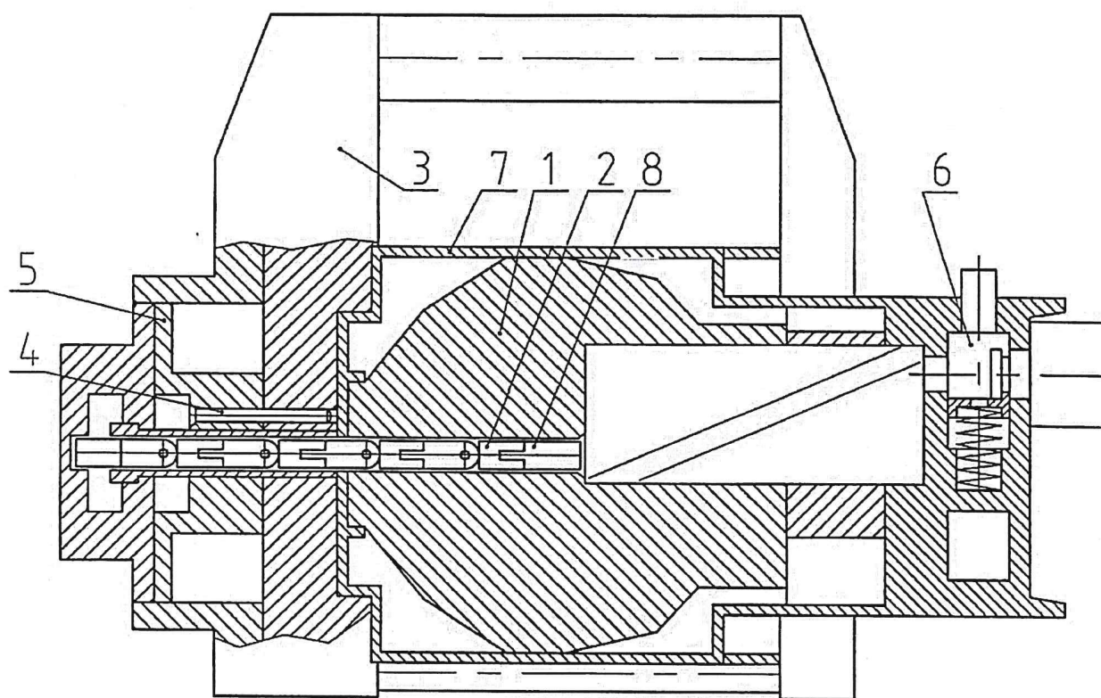
Рисунок 1. Радиационная головка гамма-дефектоскопа «Exertus Dual 120»
