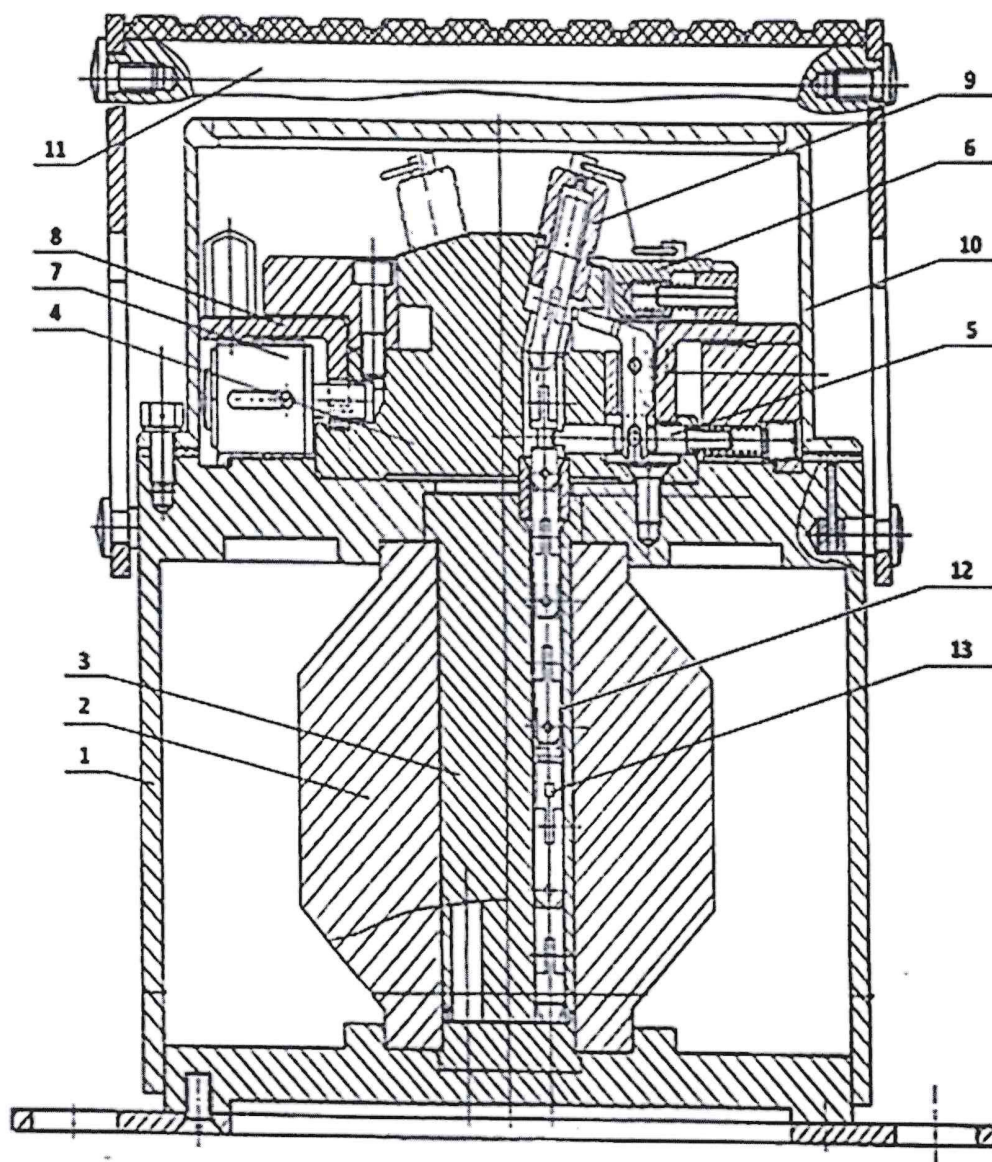
Рисунок 1 – Транспортно-перезарядный контейнер РИД-SE (RID-SE)
